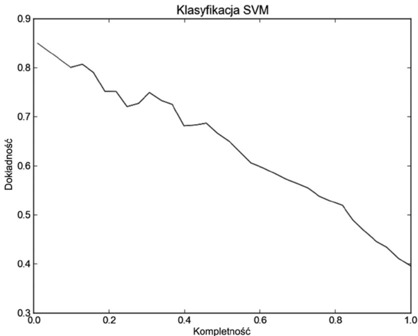
Wykres 3: Krzywa dokładności-kompletności dla klasyfikatora SVM
